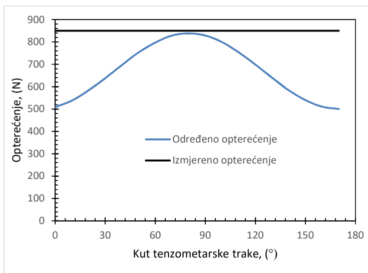
Slika 18. Utjecaj orijentacije tenzometarske trake na određivanje opterećenja
