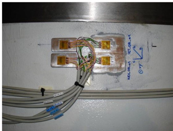
Slika 86. Mjerno mjesto na osovinskom rukavcu s prikazom postavljenih tenzometarskih traka
