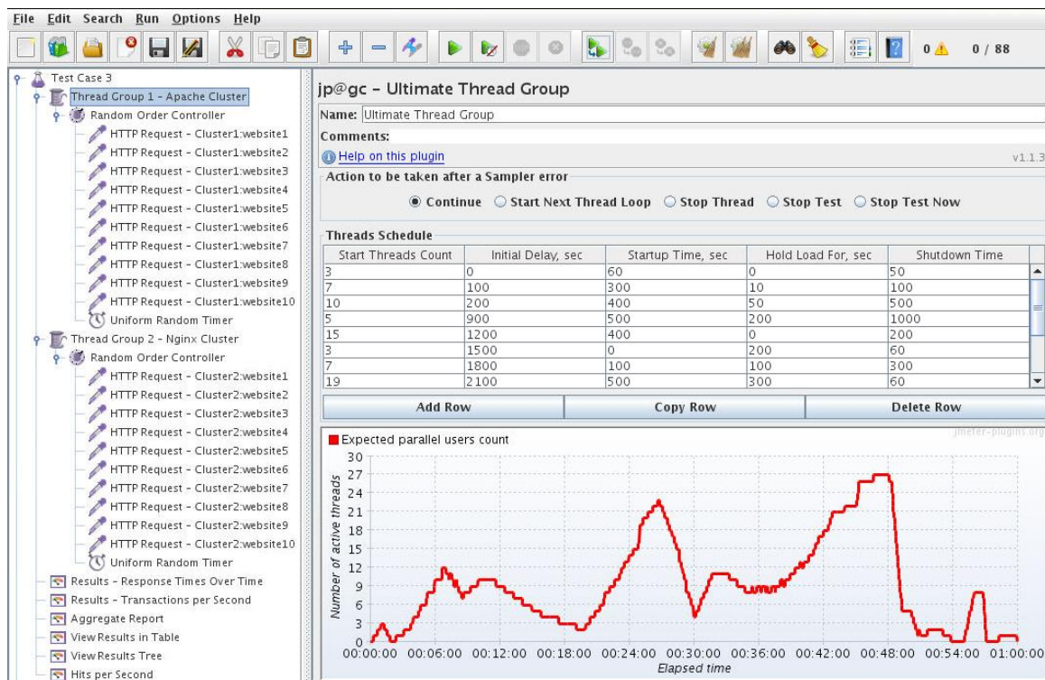
Slika 7.45. - Prikaz parametara u alatu Apache JMeter
