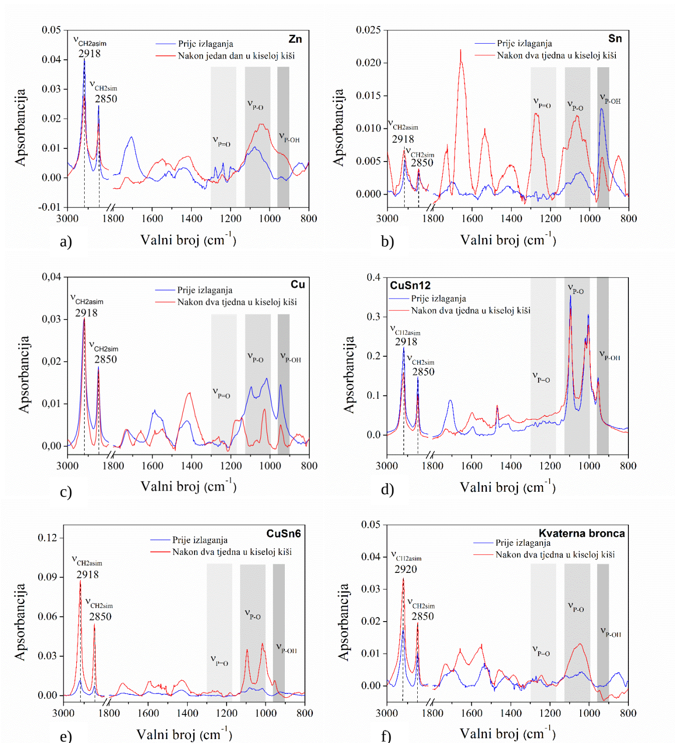
Slika 4.27. FTIR spektri COOH-PA filma na površini a) Zn, b) Sn, c) Cu, d) CuSn12, e) CuSn6 i f) kvarterne bronce. 187
