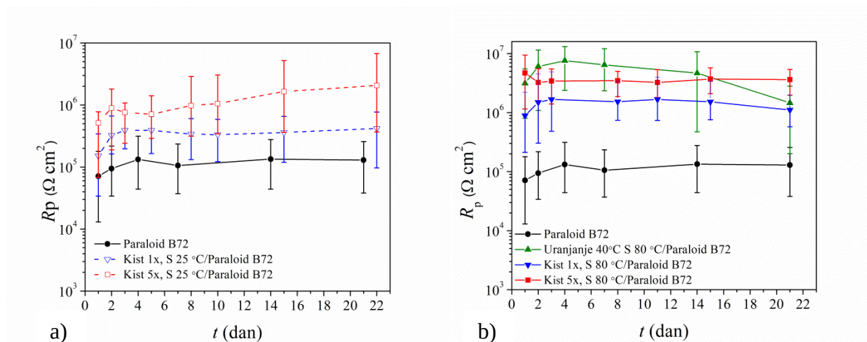
Slika 4.56. Ovisnost polarizacijskog otpora o vremenu u umjetnoj kiseloj kiši za patinirane uzorke i uzorke zaštićene Paraloidom B72 sa i bez predtretmana s COOH-PA. 82
