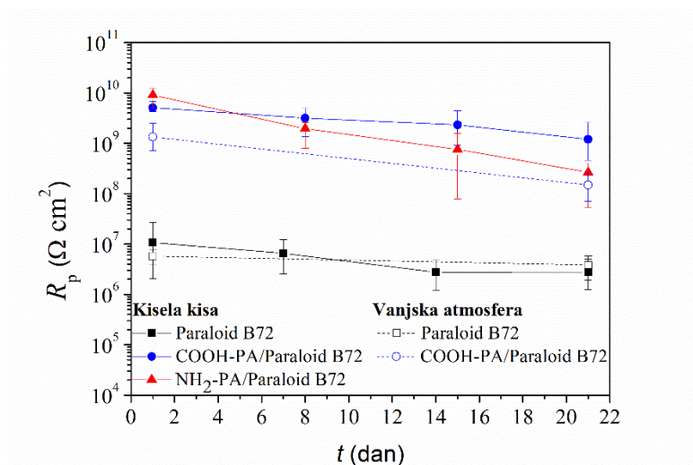
Slika 4.41. Ovisnost polarizacijskog otpora o vremenu u umjetnoj kiselj kiši i vanjskoj atmosferi za uzorke zaštićene Paraloj B72 sa i bez predtretmana s COOH-PA i NH₂-PA.
