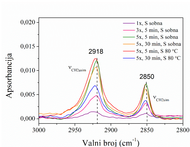
Slika 4.5. FTIR spektri filmova COOH-PA dobivenih metodom kista.
