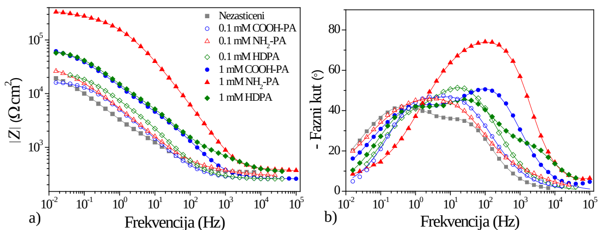
Slika 4.20. EIS – Bodeov prikaz za zaštićene uzorke prvog dana izlaganja umjetnoj kiselj kiši: a) modul impedancije i b) fazni kut (simboli – eksperimentalni podaci, linije – rezultati dobiveni korištenjem modela prikazanih na slici 4.24.). 81
