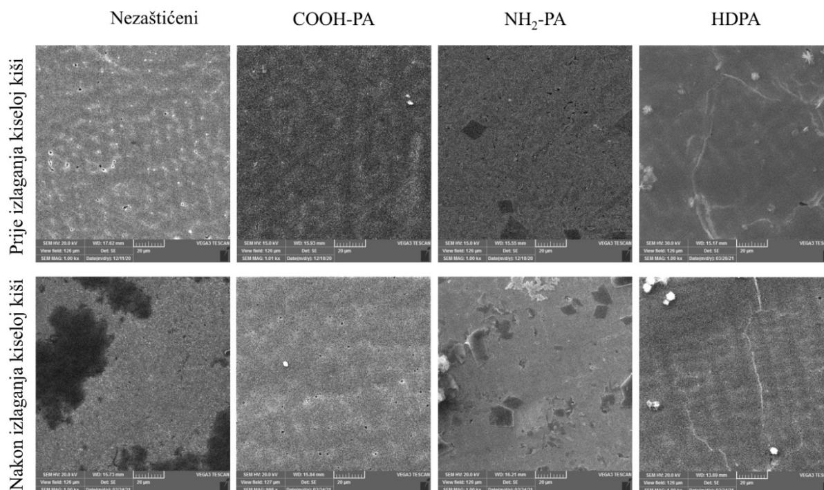
Slika 4.26. SEM slike nezaštićenog uzorka i uzoraka zaštićenih filmovima fosfonskih kiselina formiranih iz 1 mM otopina prije i nakon izlaganja umjetnoj kiseloj kiši pri povećanju od 1000x. 81
