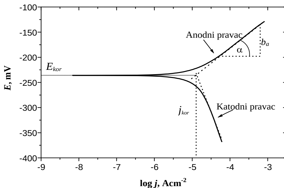
Slika 3.7. Određivanje korozijskih parametara iz polarizacijske krivulje metodom Tafelove ekstrapolacije. 2
