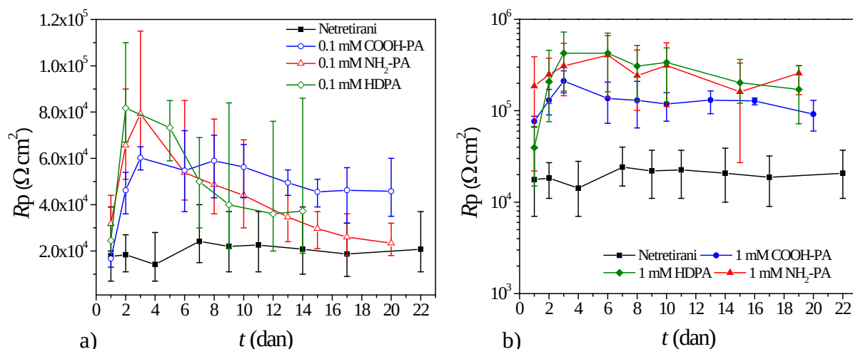
Slika 4.17. Ovisnost polarizacijskog otpora o vremenu u umjetnoj kiselj kiši za nezaštićeni uzorak CuSn12 bronce i uzorke zaštićene filmovima COOH-PA, NH 2 -PA i HDPA različitih koncentracija. 81
