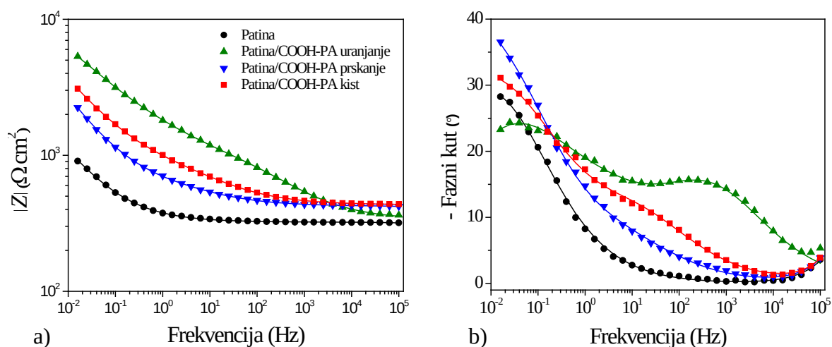
Slika 4.52 EIS – Bodeov prikaz za nezaštićeni uzorak i uzorke zaštićene filmom COOH-PA prvog dana uranjanja u kiselu kišu: a) modul impedancije i b) fazni kut (simboli – eksperimentalni podaci, linije – rezultati dobiveni korištenjem modela prikazanog na slici 4.54.). 82
