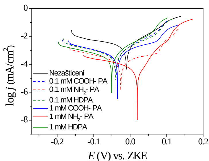
Slika 4.16. Polarizacijske krivulje dobivene u umjetnoj kiseloj kiši za nezaštićeni uzorak CuSn 12 bronce i uzorke zaštićene filmovima COOH-PA, \text{NH}_2 -PA i HDPA. 81
