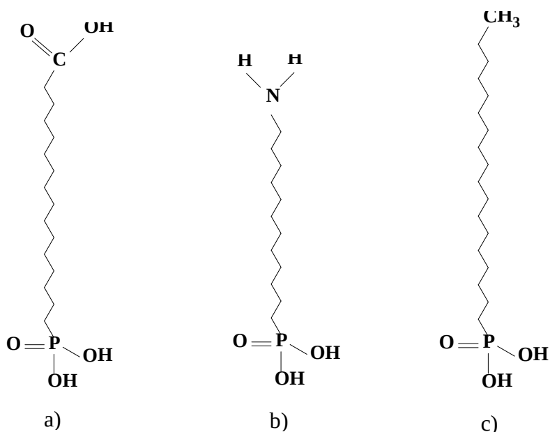
Slika 3.4. Fosfonske kiseline korištene za zaštitu bronce: a) 16-fosfonoheksadekanska (COOH-PA), b) 12-aminododecilfosfonska (NH 2 -PA) i c) heksadecilfosfonska kiselina (HDPA).
