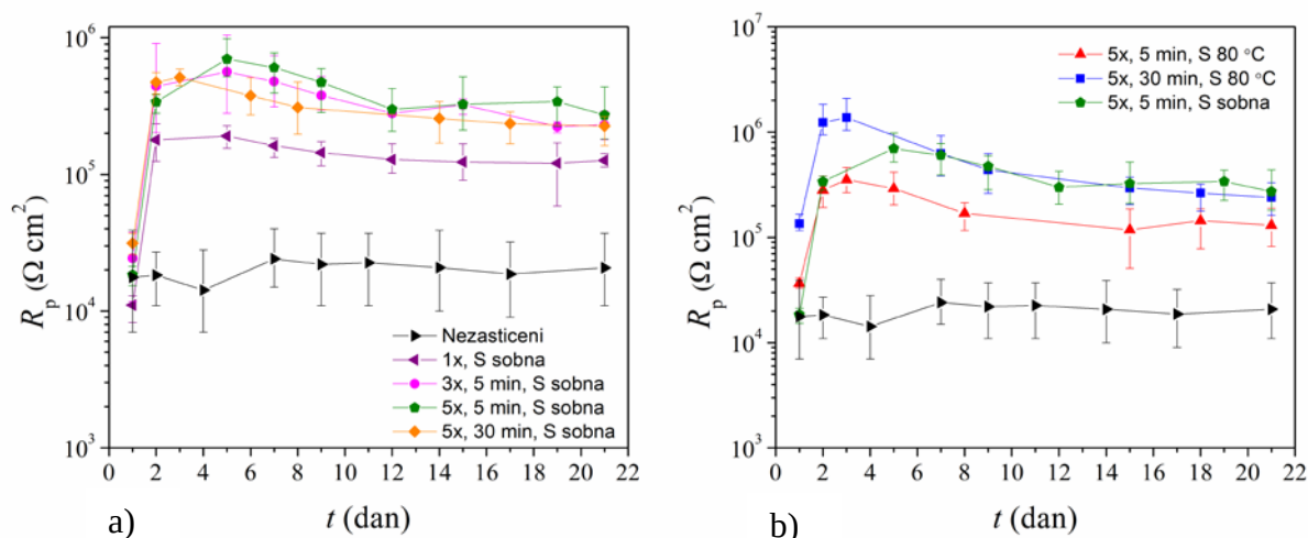
Slika 4.7. Ovisnost polarizacijskog otpora o vremenu u umjetnoj kiselj kiši za nezaštićeni uzorak CuSn12 bronce i uzorke zaštićene filmovima COOH-PA dobivenih metodom prskanja.
