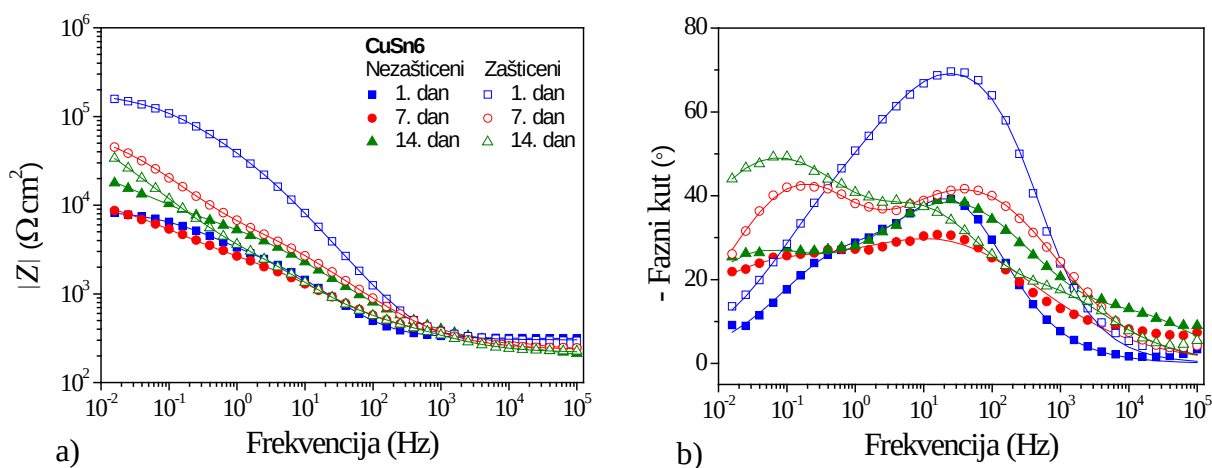
Slika 4.35. EIS – Bodeov prikaz za nezaštićeni i zaštićeni uzorak CuSn6 prvi dan, nakon tjedan dana i nakon dva tjedna izlaganja umjetnoj kiselj kiši: a) modul impedancije i b) fazni kut (simboli – eksperimentalni podaci, linije – rezultati dobiveni korištenjem modela prikazanih na slici 4.19. i 4.24.). 187
