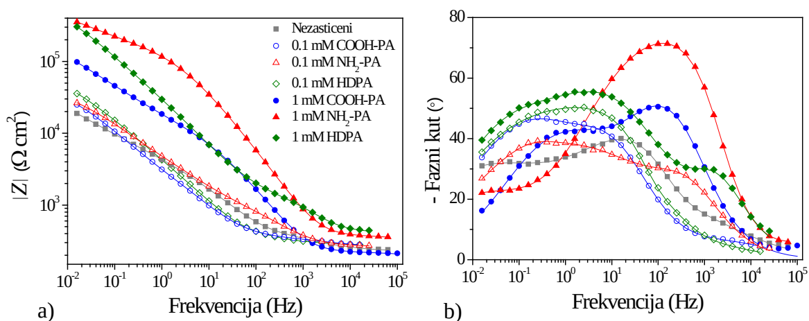
Slika 4.21. EIS – Bodeov prikaz za zaštićene uzorke nakon tjedan dana izlaganja umjetnoj kiseloj kiši: a) modul impedancije i b) fazni kut (simboli – eksperimentalni podaci, linije – rezultati dobiveni korištenjem modela prikazanih na slici 4.24.). 81
