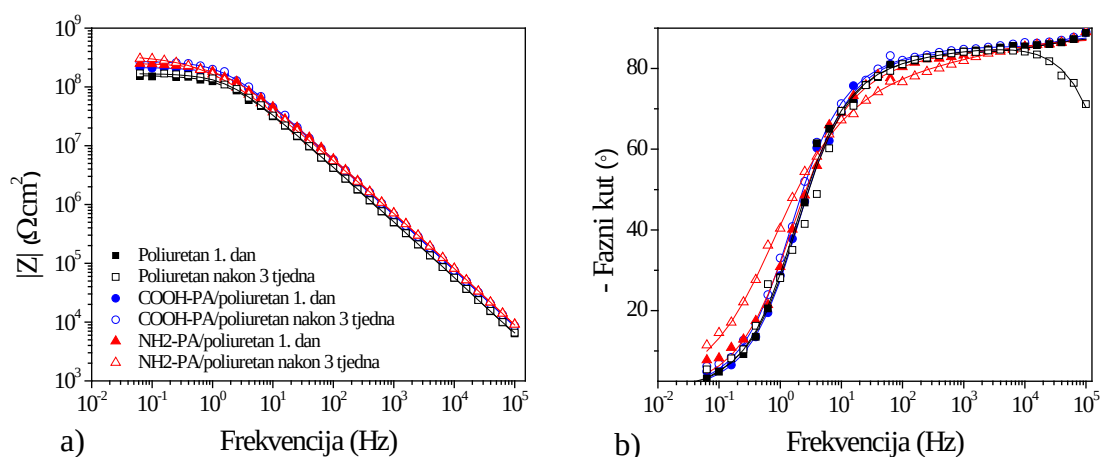
Slika 4.49. EIS – Bodeov prikaz za uzorak zaštićen poliuretanom sa i bez COOH-PA ili \text{NH}_2 -PA kao predtretmana prvi dan i nakon tri tjedna izlaganja umjetnoj kiseloj kiši: a) modul impedancije i b) fazni kut (simboli – eksperimentalni podaci, linije – rezultati dobiveni korištenjem modela prikazanih na slici 4.43.).
