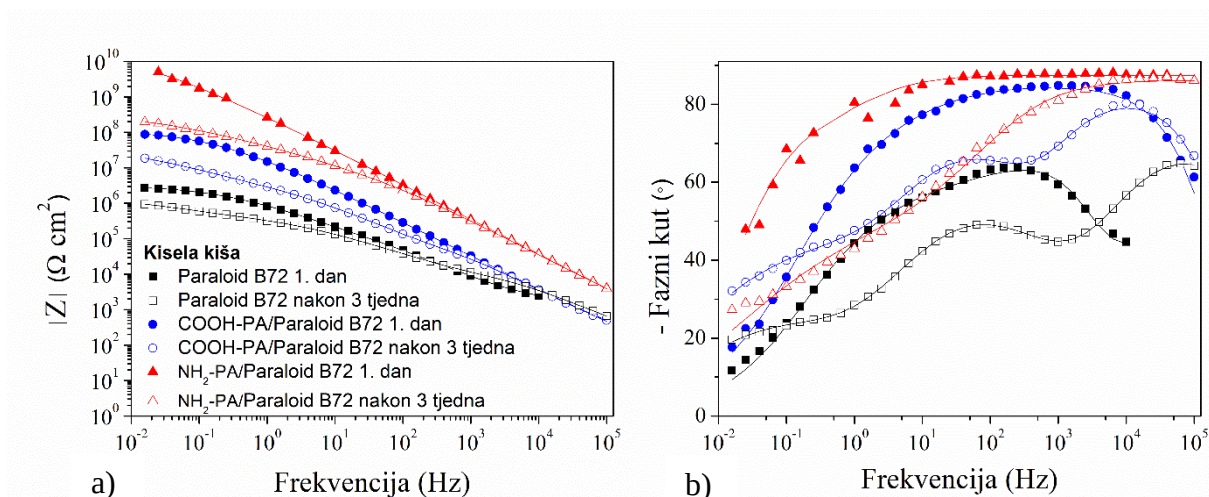
Slika 4.42. EIS – Bodeov prikaz za uzorak CuSn12 bronce zaštićen Paraloj B72 sa i bez predtretmana s COOH-PA ili NH 2 -PA, prvi dan i nakon tri tjedna izlaganja umjetnoj kiselj kiši: a) modul impedancije i b) fazni kut (simboli – eksperimentalni podaci, linije – rezultati dobiveni korištenjem modela prikazanih na slici 4.43.).
