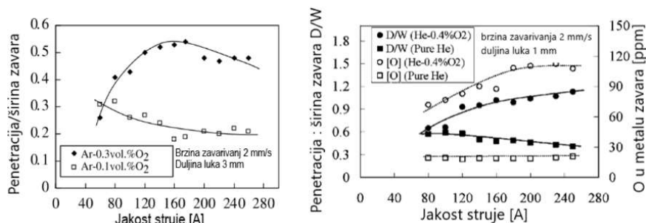
Slika 2.18 Utjecaj jaskosti struje na D/W omjer, [67] i [10]
