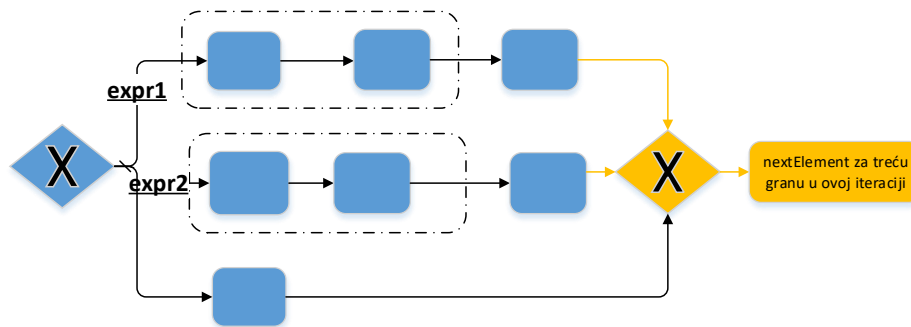
Slika 31: Vizualno - nextElements nakon izvršavanja (4)
