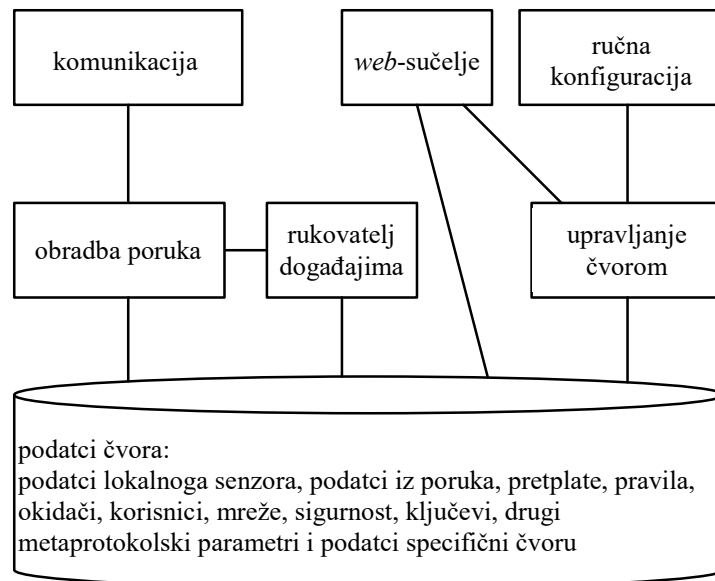
Slika 3.4. Model čvora
