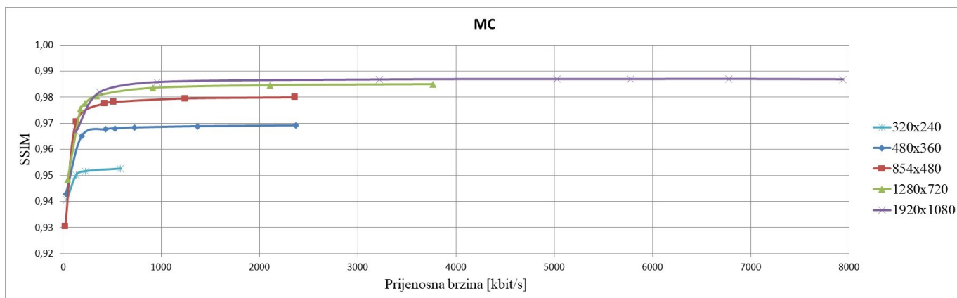
Slika 4.3. Krivulje ovisnosti SSIM-a o prijenosnoj brzini za Meridian Conversation videosignal kodiran na odabranim prostornim rezolucijama: 240p, 360p, 480p, 720p i 1080p
