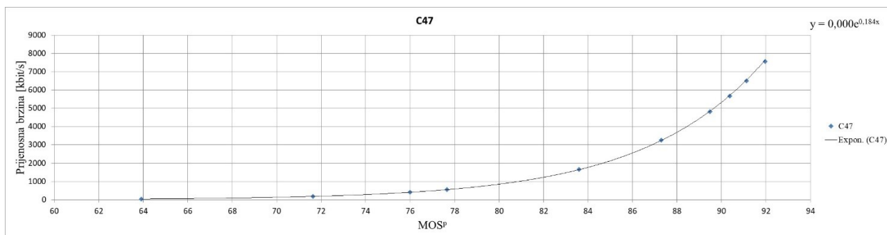
Slika 4.25. Krivulja ovisnosti prijenosne brzine o vrijednosti MOS^p Chimera1102347 (C47)
