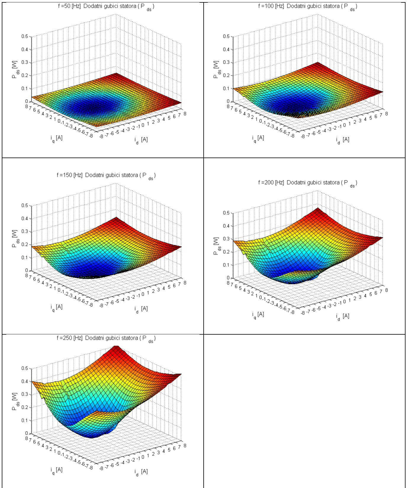
Slika C1: Dodadni gubici statora pri frekvenciji 50, 100, 150, 200 i 250 Hz
