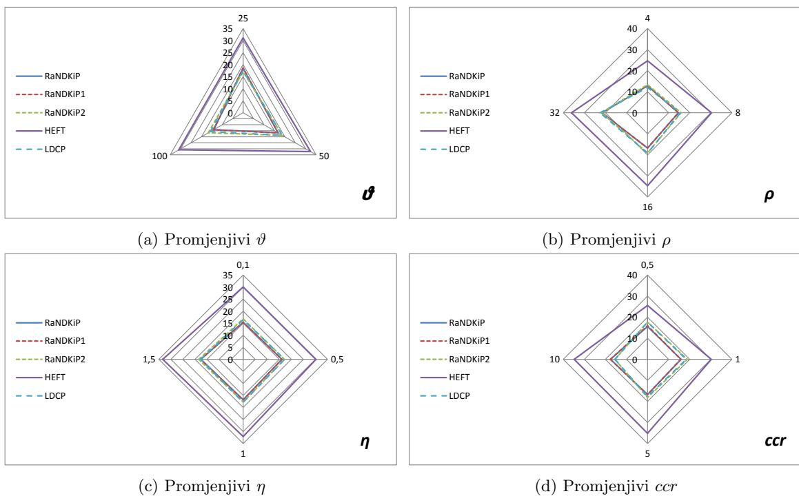
Slika 5.35: Ušteda energije kod testnih slučajeva iz repozitorija Pegasus, platforma s raznorodnom komunikacijom.
