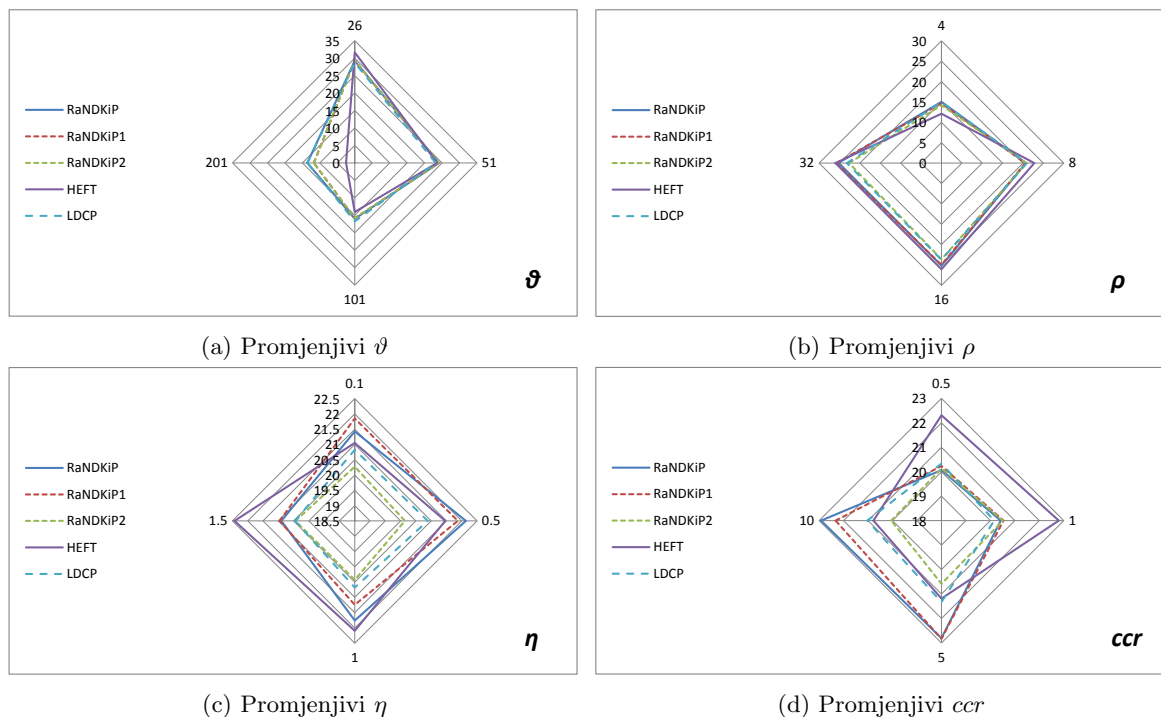
Slika 5.34: Ušteda energije kod testnih slučajeva generiranih alatom DAGGer, platforma s homogenom komunikacijom.
