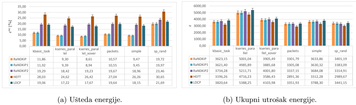
Slika 5.38: Parametri energije u sustavu s raznorodnom komunikacijom platforme za različite strukture programa generiranih alatom TGFF.
