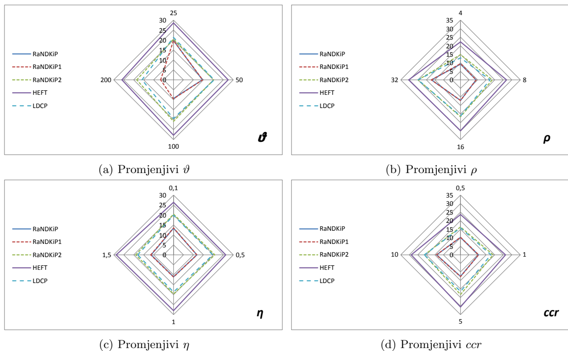
Slika 5.37: Ušteta energije kod testnih slučajeva generiranih alatom TGFF, platforma s raznorodnom komunikacijom.
