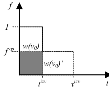
Slika 4.15: Primjer skaliranja frekvencije za obradbeni isječak.
