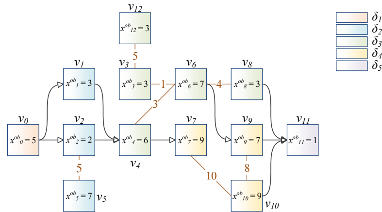
Slika 4.3: Model programa.
