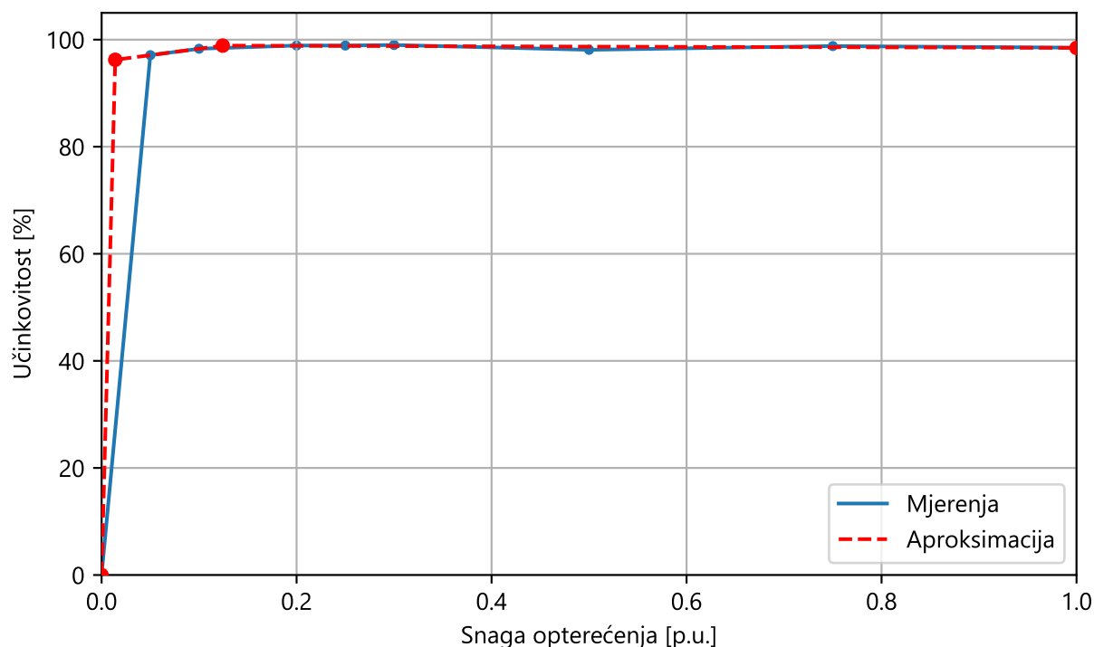
Slika 5.7: Linearna aproksimacija nelinearne karakteristike učinkovitosti izmjenjivača SMA Sunny Highpower Peak3 SHP 150-20 pri različitim opterećenjima korištena za referentni slučaj
