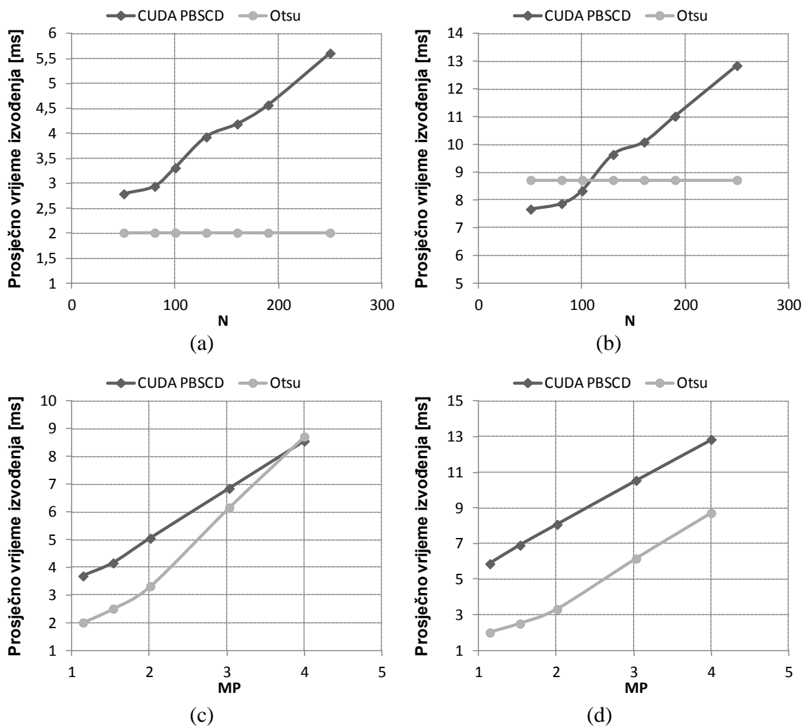
Slika 4.29: Prosječno vrijeme izvođenja u 100 iteracija CUDA PBSCD i Otsu metode: (a) slika veličine 1038 \times 1098 pikseli i promjenjivi N , (b) slika veličine 1946 \times 2054 pikseli i promjenjivi N , (c) N = 120 i promjenjiva veličina slike izražena u megapikselima (MP), (d) N = 250 i promjenjiva veličina slike u MP.
