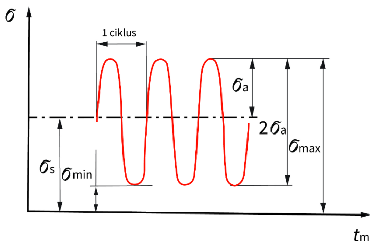
Slika 1.4. Ciklusi napreznja
