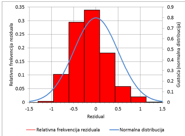
Slika 7.19 Histogram reziduala
