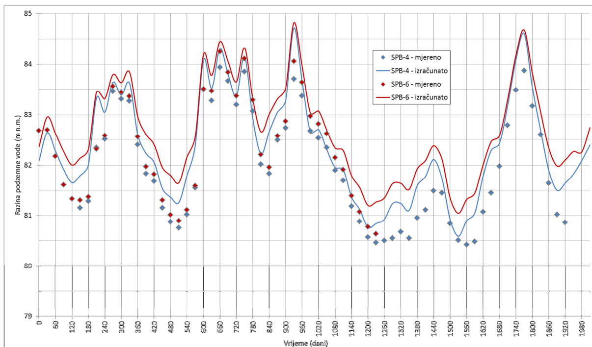
Slika 7.12 Nivoigrami kalibracije modela za piezometre SPB-4 i SPB-6
