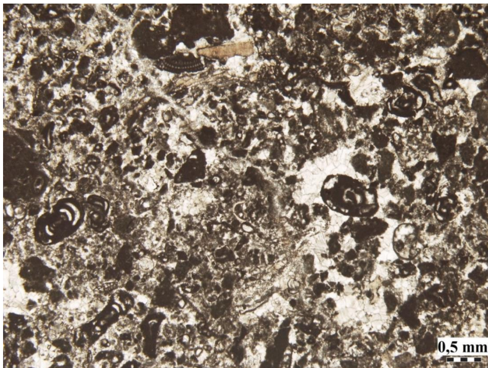
Slika 5.20. Mikrofacies skeletnog vekstona–pekstona srednjeg do gornjeg cenomana; uzorak ĆV-7 ( 45^{\circ}29'50.7''N , 14^{\circ}2'3.8''E ).
