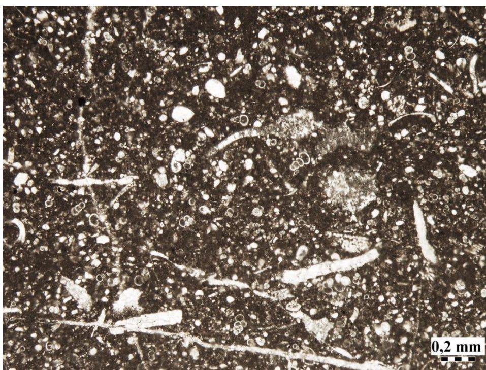
Slika 5.25. Mikrofacijes bioklastičnoga vekstona–pekstona litostratigrafske jedinice Sv. Duh s kalcisferulidama, planktonskim foraminiferama te bioklastima bodljikaša; uzorak L-35 (45°27'4.2"N, 14°3'37.5"E).
