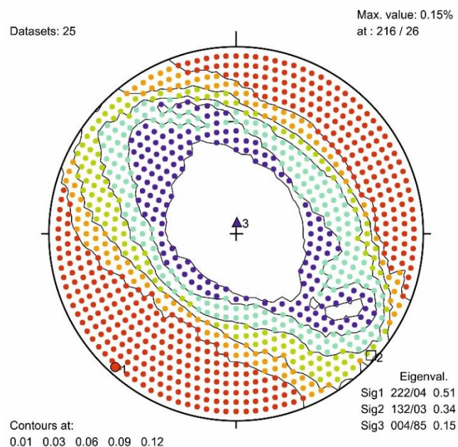
Slika 5.54. Strukturni dijagram pravih diedara za grupu reverznih rasjeda RR-1 s izračunom osi paleonapreznosti – najveća ( \sigma_1 ), srednja ( \sigma_2 ) i najmanja os paleonapreznosti ( \sigma_3 ).
