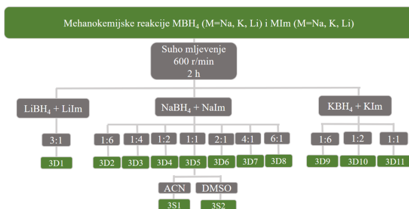
Shema III. Mehankemijske reakcije monometalnih alkalijskih borohidrida i alkalijskih imidazolata.
