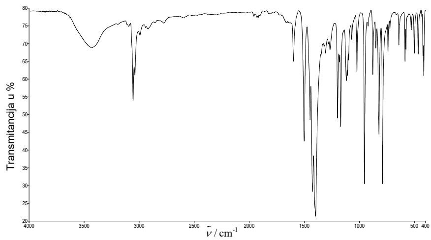
Prilog 2. FT-IR spektar spoja 2.
