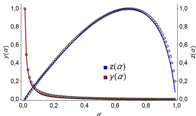
Slika 82. Teorijske y(\alpha) i z(\alpha) vrijednosti za reakciju nastajanja azodioksida spoja 3 prikazane su crnim kružićima, dok su eksperimentalne vrijednosti prikazane crvenom, odnosno plavom krivuljom. Teorijske vrijednosti računane su s pretpostavkom modela Šestáka i Berggrena definiranog parametrima n = 0,6 ; m = 0 ; p = -1 .
