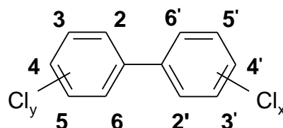
Slika 2.4. Opća strukturalna formula polikloriranih bifenila
