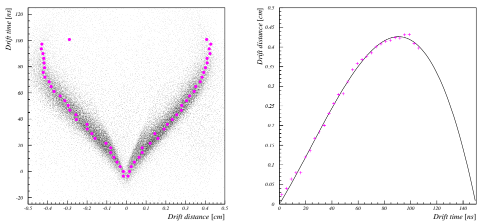
SLIKA 3.3: TIPIČNA OVISNOST DRIFTNE UDALJENOSTI O DRIFTNOM VREMENU RAVNINA ENGE DRIFTNE KOMORE. Lijevo ODREĐIVANJE TOČAKA ZA KALIBRACIJU. Desno ODREĐIVANJE MAPE DRIFTNO VRIJEME-POZICIJA PRILAGODBOM OVISNOSTI DRIFTNE UDALJENOSTI O DRIFTNOM VREMENU POLINOMOM TREĆEG STUPNJA.
