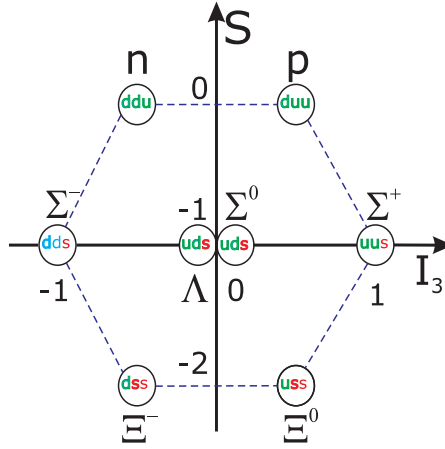
SLIKA 1.1: OKTET LAKIH J^P=1/2^+ BARIONA. PRIKAZ OVISNOSTI O TREĆOJ KOMPONENTI IZOSPINA I_3 I STRANOSTI.
