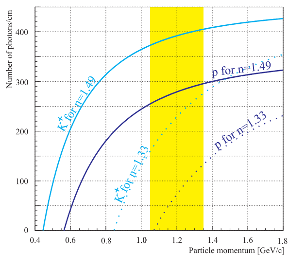
SLIKA 2.13: OVISNOST BROJA PRODUCIRANIH FOTOELEKTRONA U ČERENKOVLEJIM DETEKTORIMA O IMPULSU KAONA I PROTONA ZA DVA RAZLIČITA RADIJATORA: VODA ( n=1.33 ) I AKRILNI RADIJATOR ( n=1.49 ). OBOJANO PODRUČJE REPREZENTIRA IMPULSNU AKCEPTANCIJU HKS-A.
