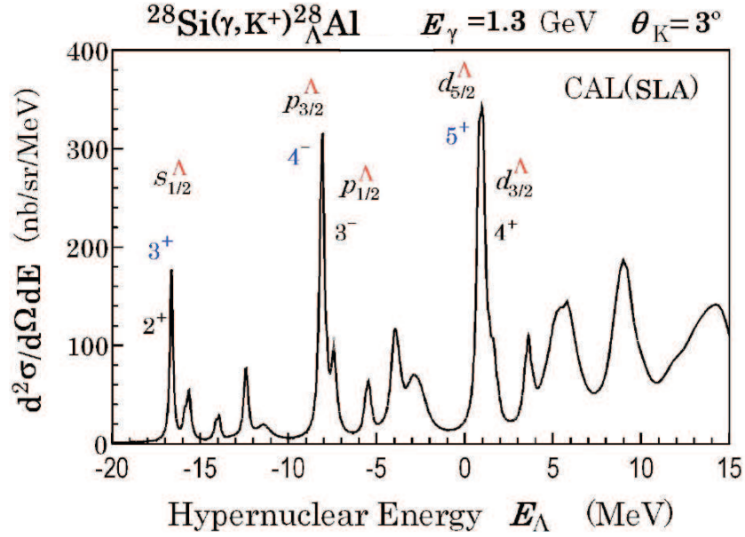
SLIKA 5.7: TEORIJSKI PREDVIĐEN SPEKTAR ZA ^{28}\text{Si}(e, e'K^+)_{\Lambda}^{28}\text{Al} REAKCIJU. RAČUN JE RAĐEN S E_{\gamma} = 1.3 \text{ GeV} I \theta_{K^+}^{LAB} = 3^\circ U SLA IZOBARNOM MODELU [31] [33].
