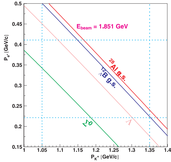
SLIKA 2.2: KORELACIJA MOMENATA DETEKTIRANIH RASPRŠENIH ELEKTRONA I KAONA. RAČUN JE NAPRAVLJEN SA: E_e = 1.851 GeV, PRETPOSTAVLJENIM ENERGIJAMA VEZANJA {}^{12}_{\Lambda}B OSNOVNOG STANJA OD -11.37 MeV [27] I {}^{28}_{\Lambda}Al STANJA OD -16.92 MeV [19] .)
