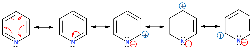
Shema 2. Rezonantne strukture piridina.
