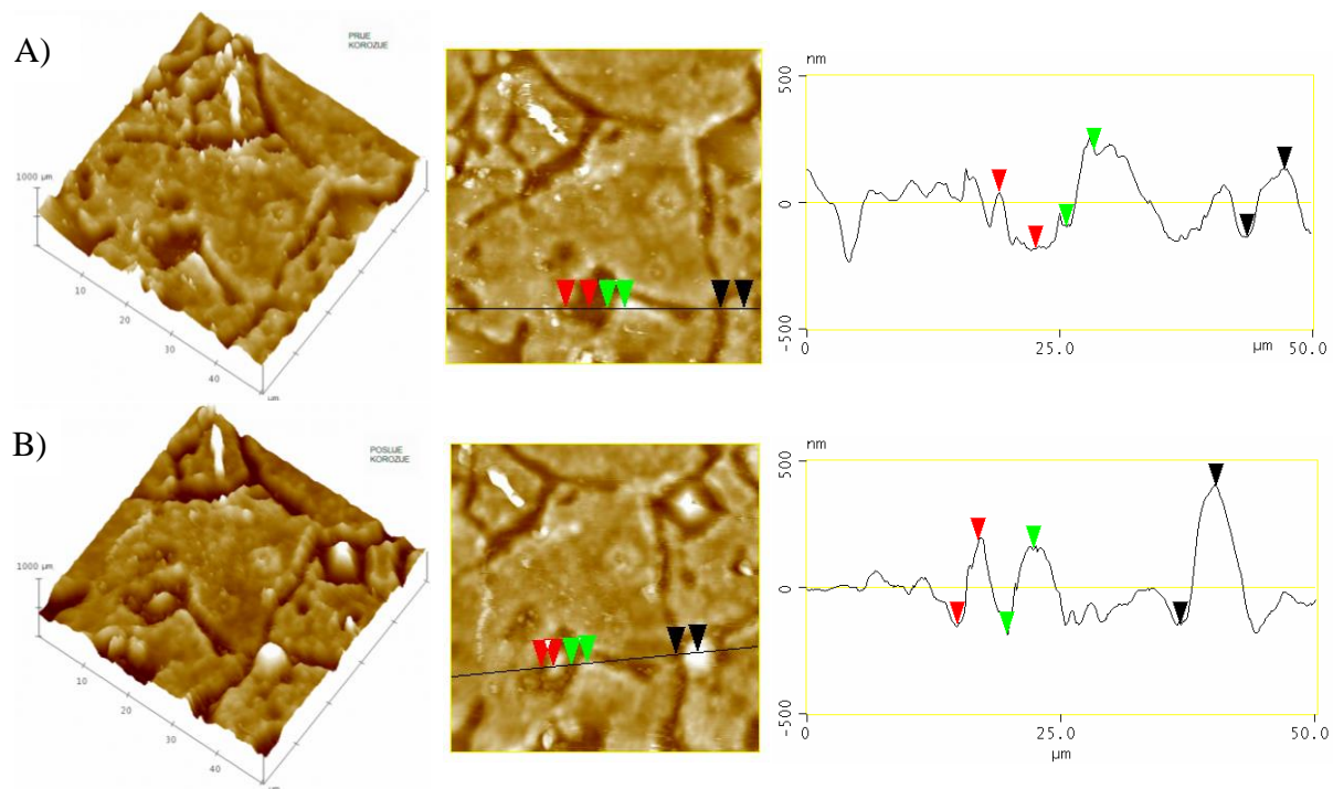
Slika D14. 3-D i 2-D AFM snimke površine i analiza presjeka sol-gel 5YSZ filma s tri sloja (600 °C, zrak) kod povećanja 50 \mu\text{m} \times 50 \mu\text{m} : A) prije korozije i B) nakon korozije.
