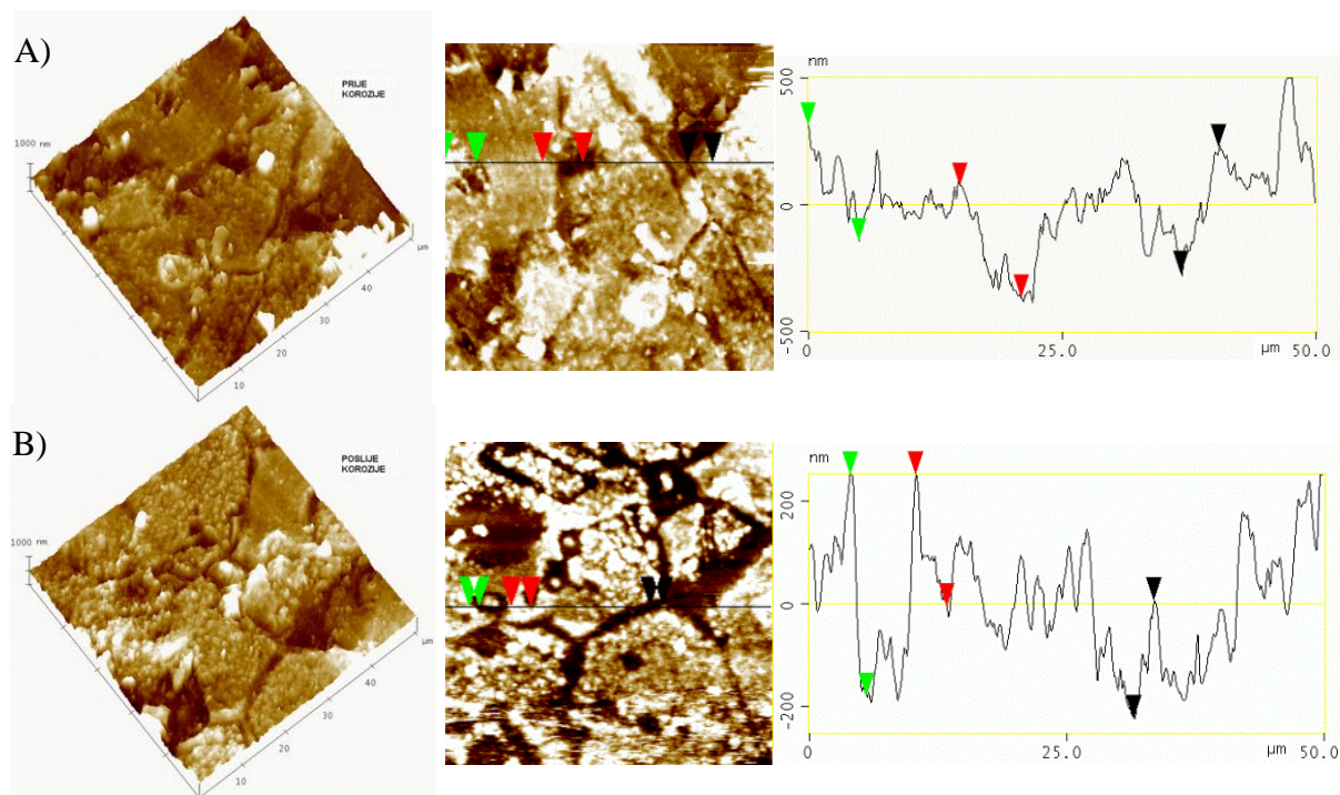
Slika D13. 3-D i 2-D AFM snimke površine i analiza presjeka sol-gel 5YSZ filma s jednim slojem (600 °C, zrak) kod povećanja 50 \mu\text{m} \times 50 \mu\text{m} : A) prije korozije i B) nakon korozije.
