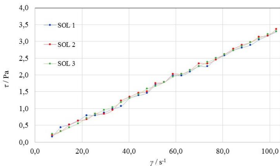
Slika 40. Ovisnost smičnog napreznjanja ( \tau ) o brzini smicanja ( \dot{\gamma} ) svježe pripremljenih solova. SOL 1 (3 mol% Y 2 O 3 ), SOL 2 (5 mol% Y 2 O 3 ) i SOL 3 (7 mol% Y 2 O 3 ).
