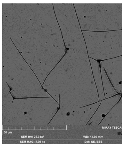
Slika 90. SEM slika površine uzorka nehrđajućega čelika AISI 316L prevučenog troslojnim 5YSZ filmom toplinski obrađenim u vakuumu na 600 °C, pri povećanju 200×.
