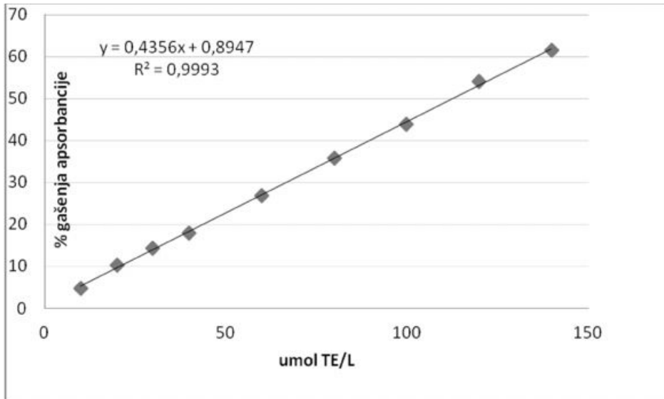
Slika 7. Baždarni dijagram
