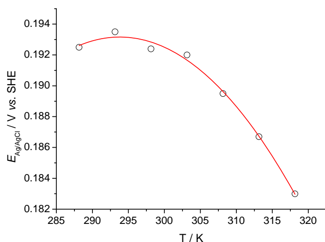
Slika 4.92. Temperaturna ovisnost potencijala Ag/AgCl elektrode prema SHE: pH = 7,5, [NaH 2 PO 4 ] = 50 mM, [NaCl] = 0,1 M.
