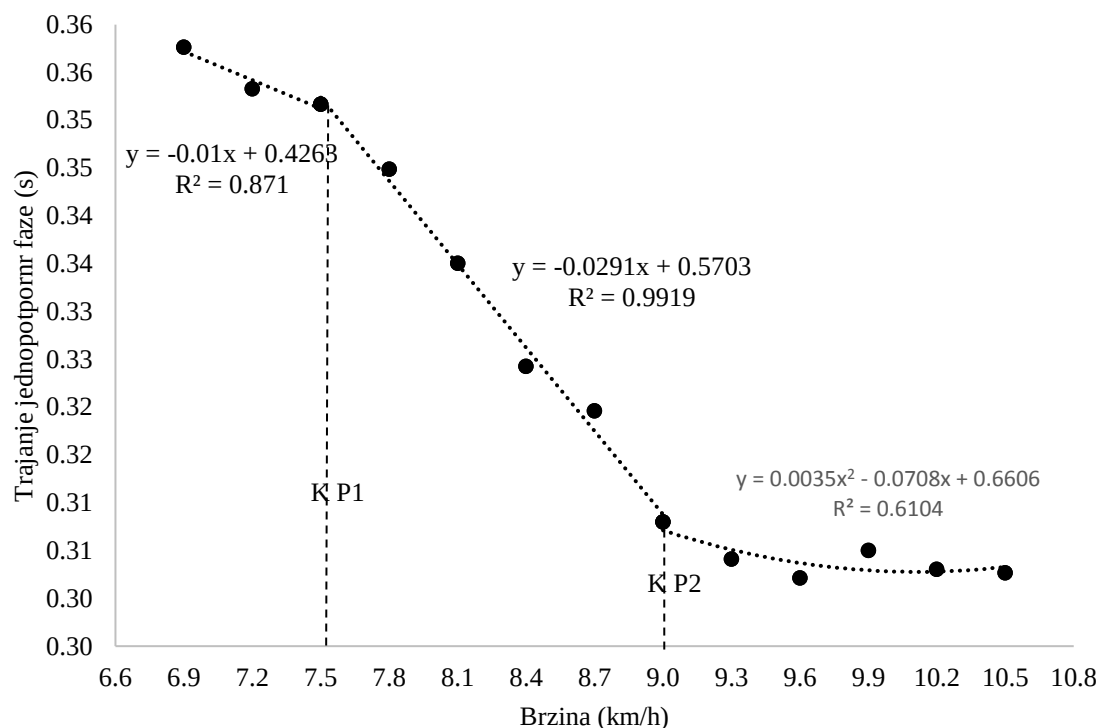
Slika 4.5.2.1. Prikaz PRVOG modela kretanja trajanja jednogpotpurne faze u testu T03 – tri zone: 1. linearan pad – 2. linearan pad – 3. polinom 2. stupnja (primjer ispitanika br. 21)
