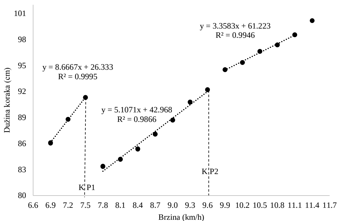
Slika 4.5.1.3. Prikaz TREČEG modela kretanja dužine koraka u testu T03 – tri zone: 1. linearan porast – 2. pad + linearan porast – 3. linearan porast (primjer ispitanika br. 14)
