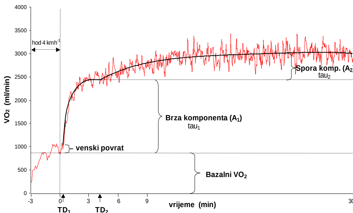
Slika 1.4.1. Kinetika \text{VO}_2 , A_1 i A_2 su brza i spora komponenta, \text{TD}_1 i \text{TD}_2 su odgovarajuća vremena odgode, \tau_1 i \tau_2 su odgovarajuće vremenske konstante (Šentija, 2002).
