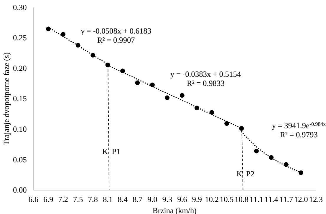
Slika 4.5.3.1. Prikaz modela kretanja trajanja dvopotpore faze u testu T03 – tri zone: 1. linearan pad – 2. linearni pad – 3. eksponencijalan pad (primjer ispitanika br. 9)
