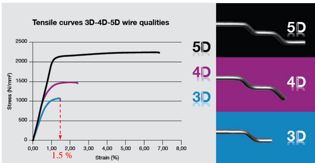
Slika 3.2 Dijagram naprežanje-deformacija za Dramix vlakna s različitim oblikom kuka
