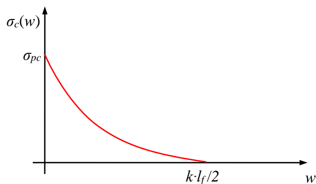
Slika 2.17 Veza vlačno naprezanje kompozita-širina pukotine ( \sigma_c-w )
