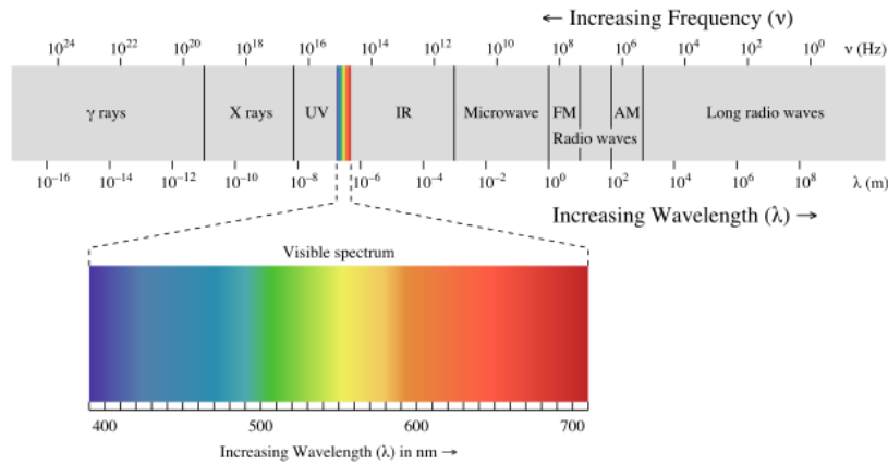
Figure 10: EM spectrum 3
