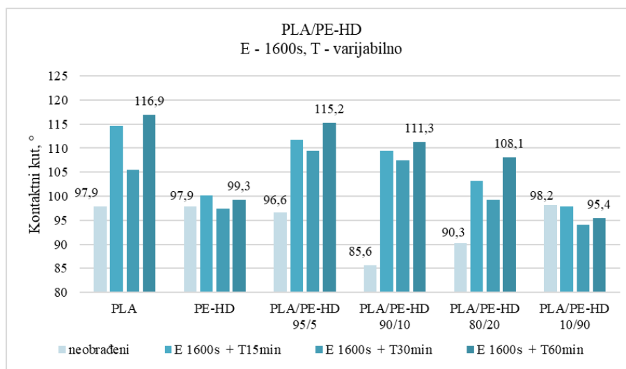
Slika 54. Izmjereni kontaktni kutovi kod polimernih mješavina PLA/PE-HD pripremljenih u ekstruderu pri različitim uvjetima obrade CF x -om (E – jetkanje; T – prevlačenje CF x -om)
