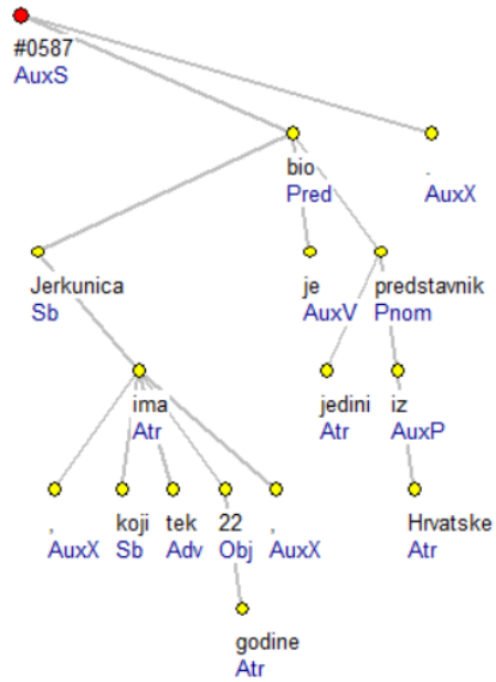
27. slika: Atributna rečenica u prvoj inačici HOBIS-a (Tadić 2007).
