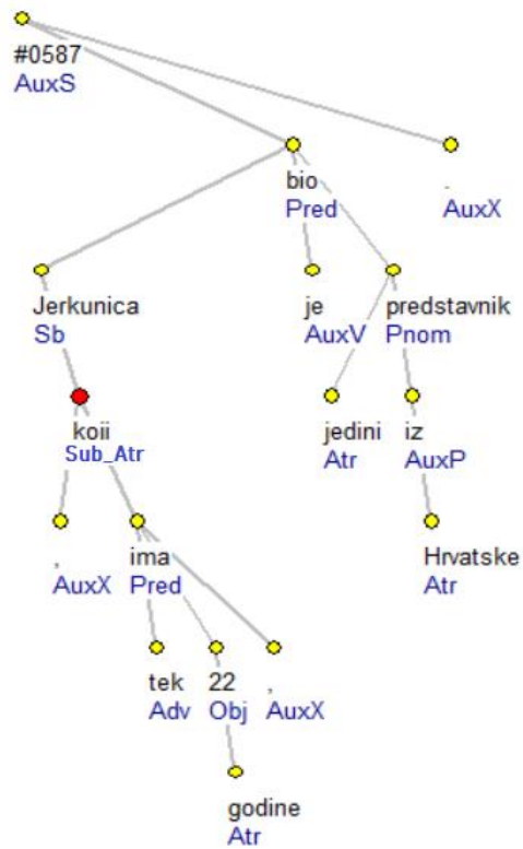
28. slika: Atributna rečenica u HOBIS-u 2.0.
