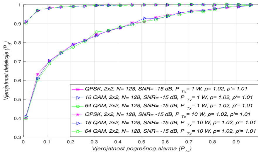
Slika 7.10. Krivulje radnih karakteristika prijelnika (ROC krivulje) ostvarene s metodom detekcije energije (ED) za MIMO sustav pod utjecajem različitih snaga odašiljanja ( P_{Tx} ) primarnog korisnika (PU) i modulacijskim shemama
