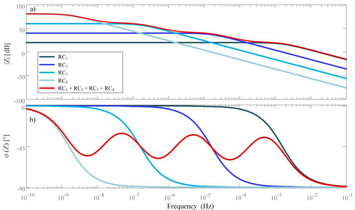
Slika 3.5: Ilustracija modeliranja CPE-a pomoću četiri serijski spojena paralelna RC člana.
