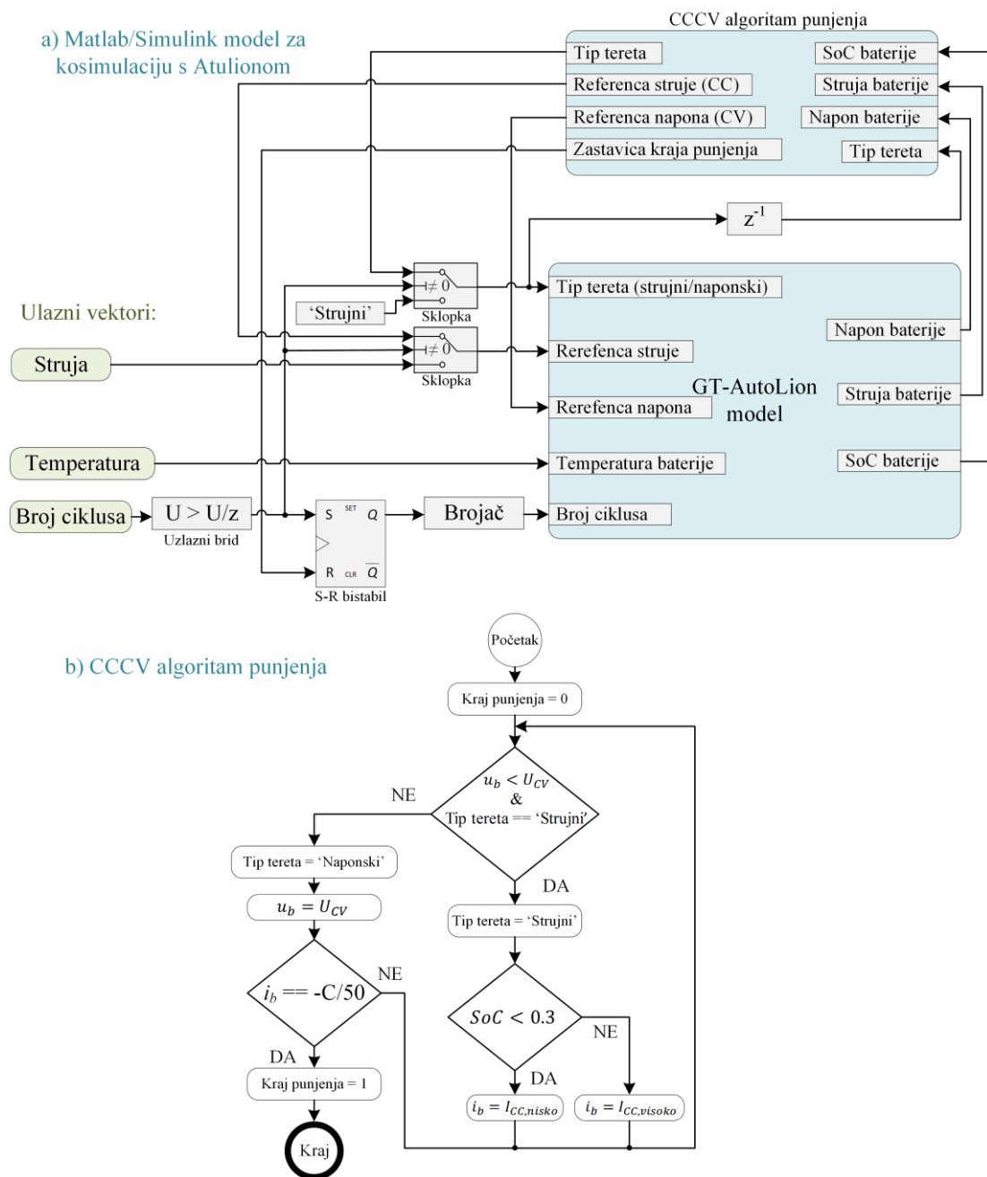
Slika 4.8: a) Ilustracija Matlab/Simulink modela za kosimulaciju s Autolion modelom ćelije, te b) implementirani algoritam CCCV punjenja.
